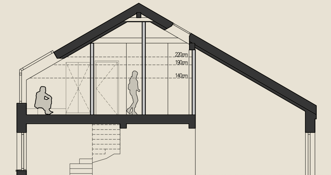
PRZEKRÓJ PRZEZ ANTRESOŁĘ
